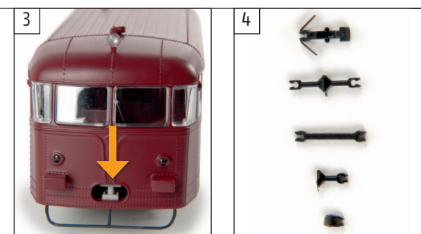
Der Kupplungs-Satz (5 Varianten) ist als Ersatzteil unter der Art.: 10152 separat erhältlich.
